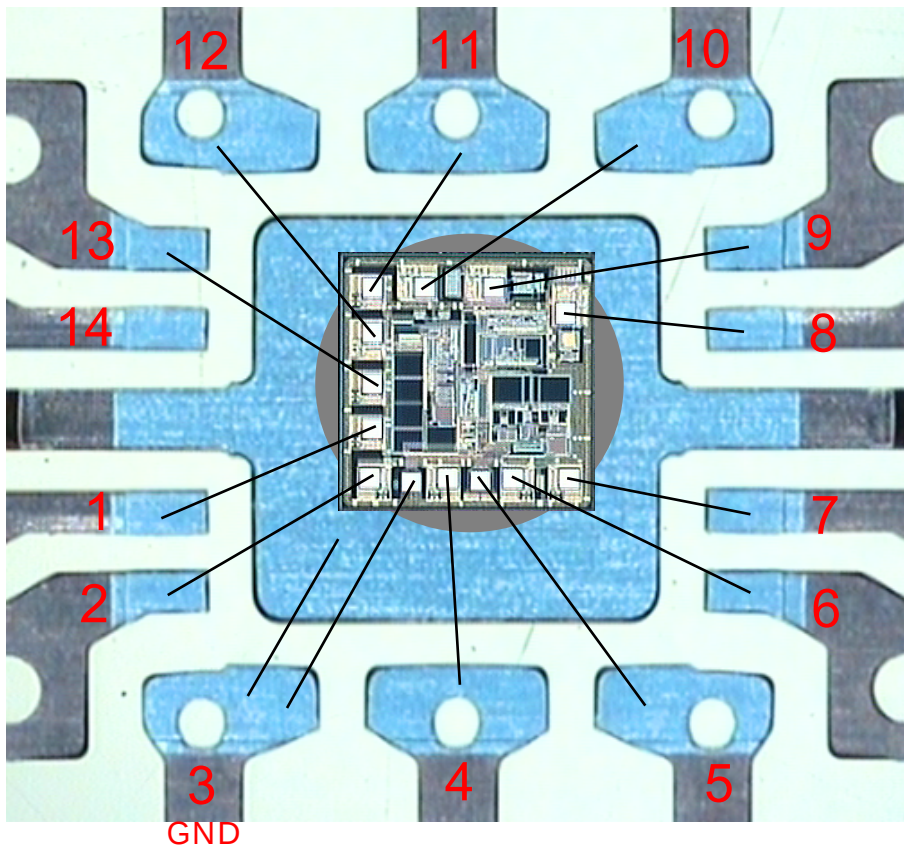
焊线示意图(Bonding Diagram)
